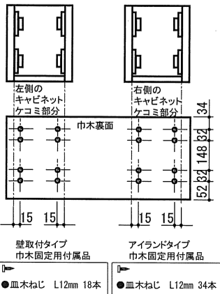
【巾木固定金具取付位置】
