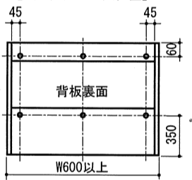
【壁面固定用下穴位置】
