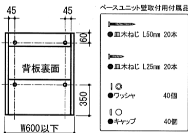
【アイランド床固定用下穴位置(参考)】
