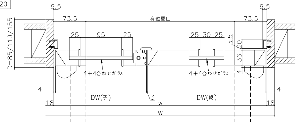
詳細図 1/4
