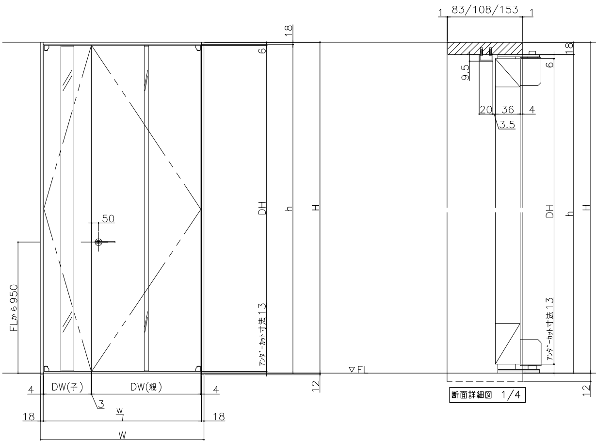
正面図 1/20
