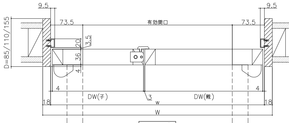
詳細図 1/4
