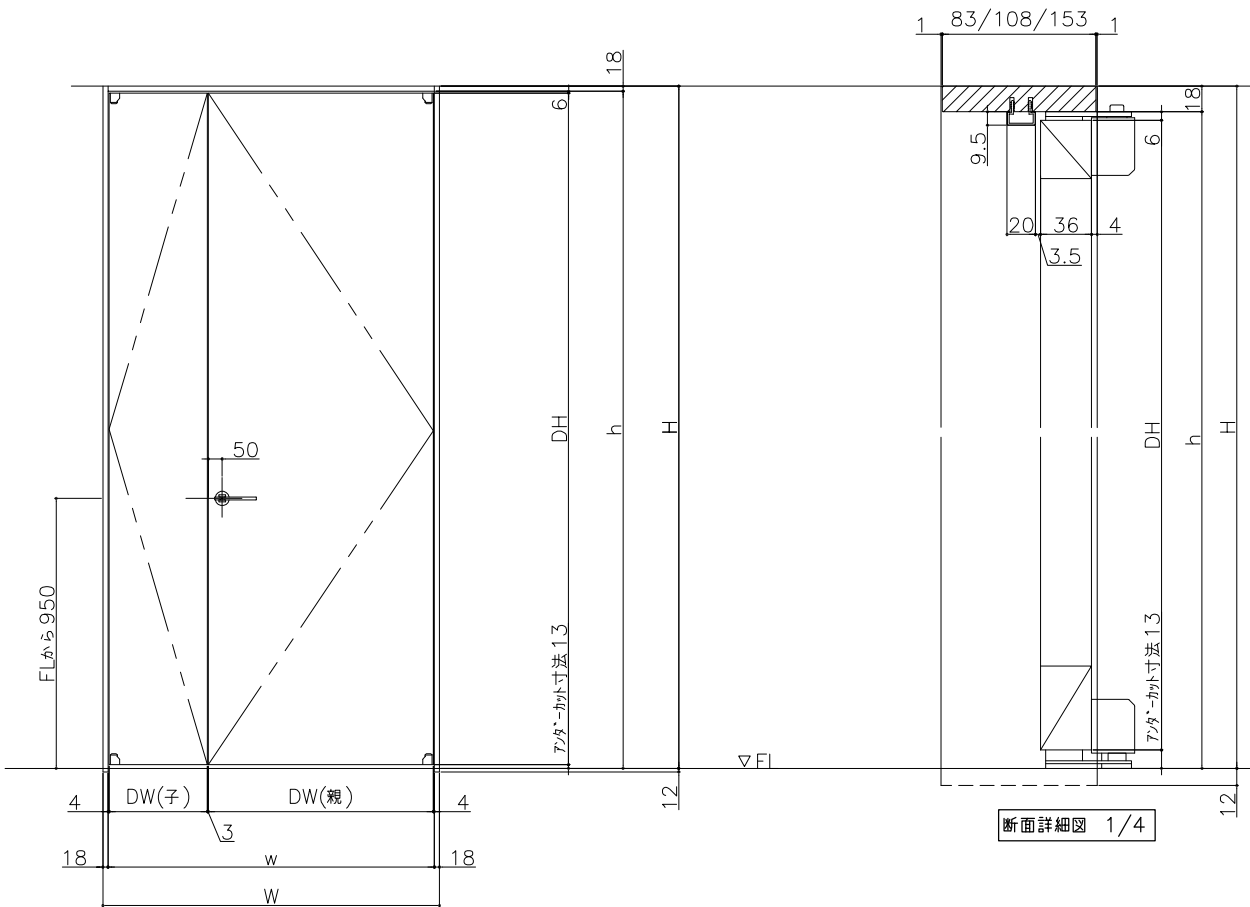
正面図 1/20
