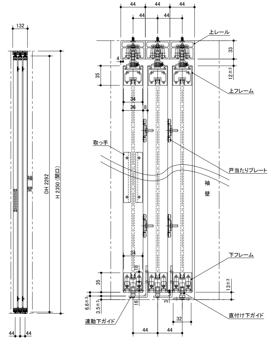
詳細図 1/2
