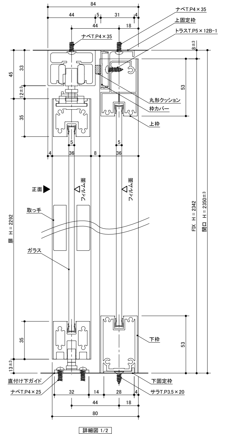
詳細図 1/2
