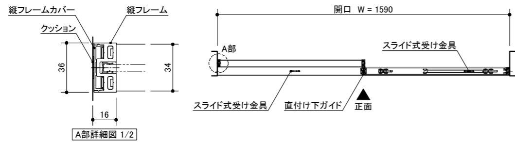
A部詳細図 1/2
