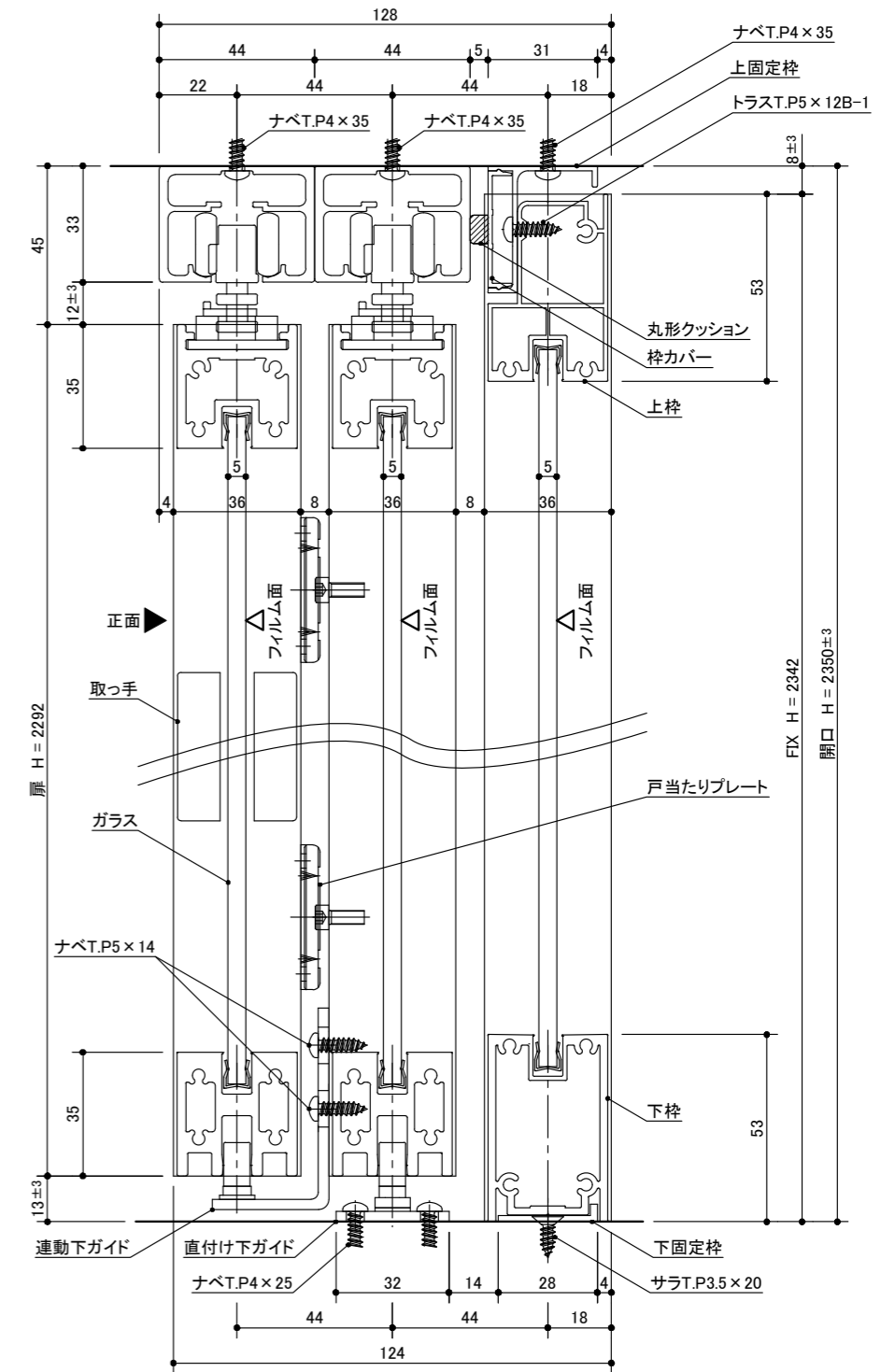
詳細図 1/2
