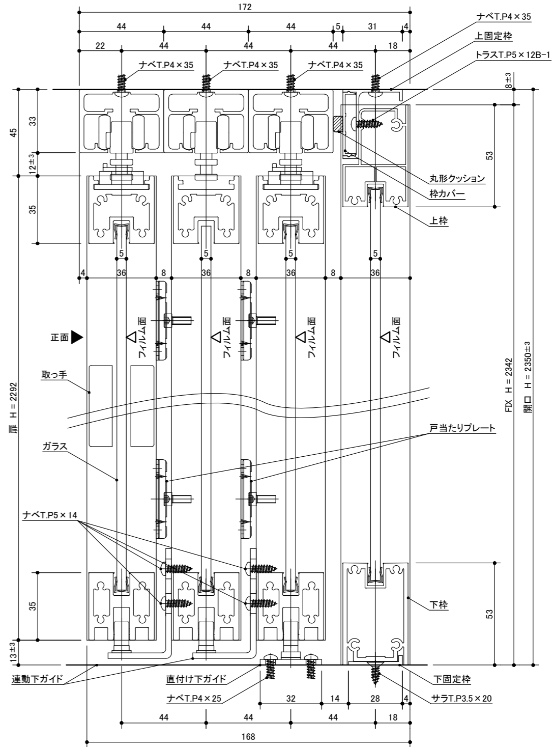
詳細図 1/2
