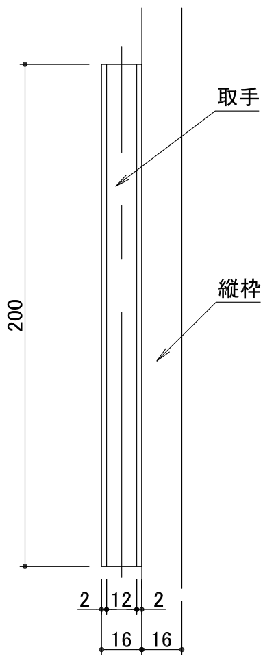
正面図
