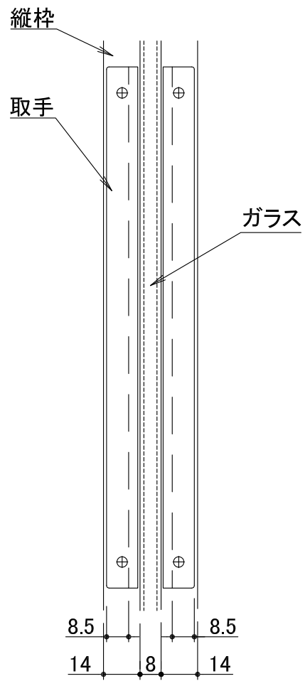
側面図
